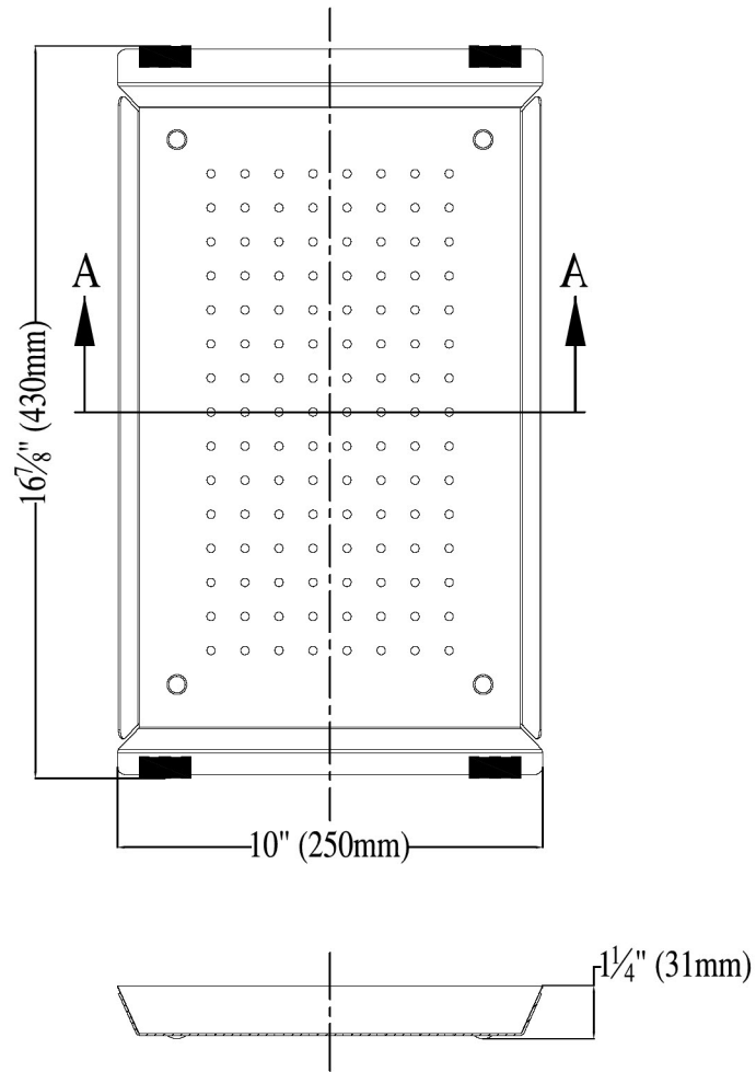
SECTION A-A
